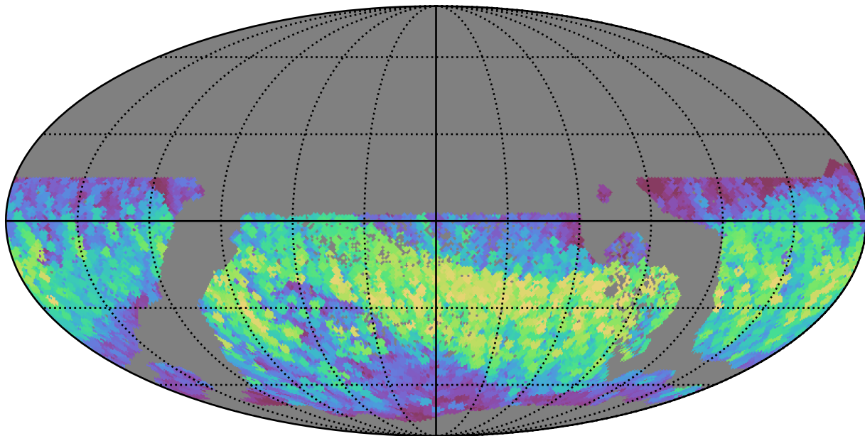
all_long_v3.4_10yrs WFD i band: Max normairmass
