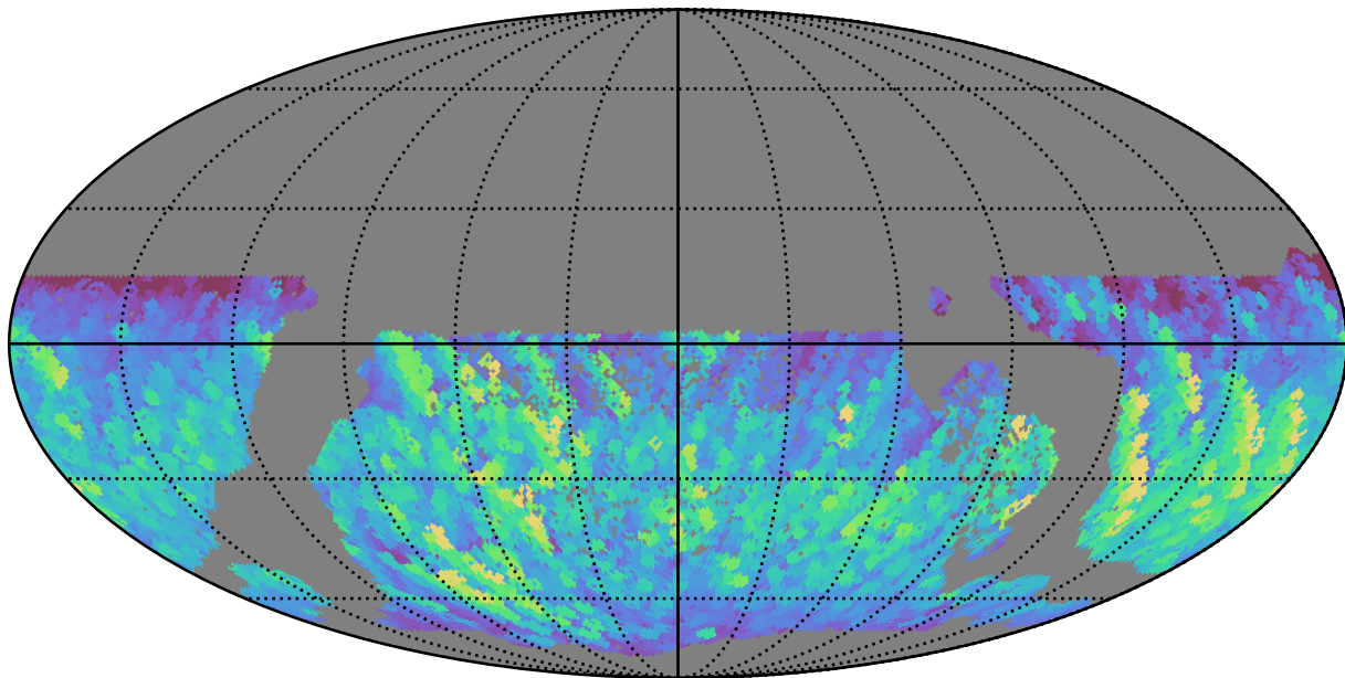
all_long_v3.4_10yrs WFD g band: Max normairmass
