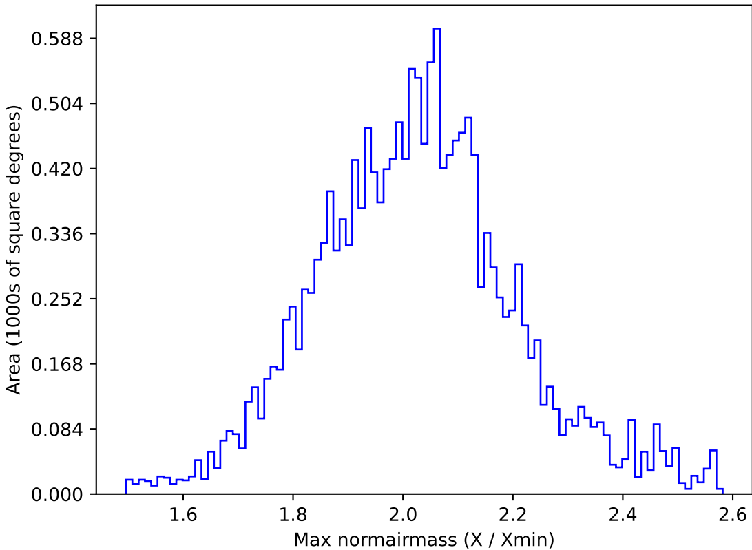
all_long_v3.4_10yrs WFD g band: Max normairmass
