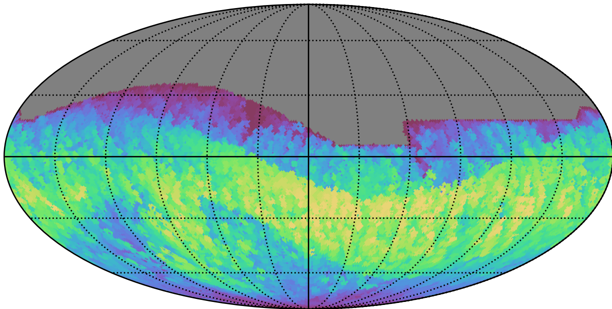
all_long_v3.4_10yrs All sky z band: Max normairmass
