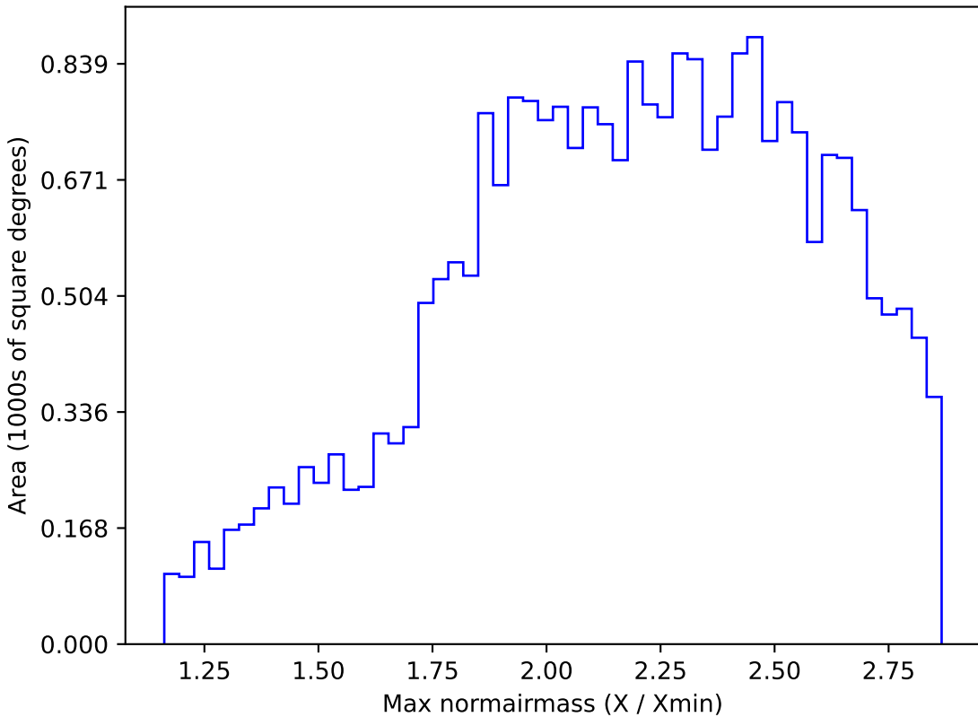
all_long_v3.4_10yrs All sky z band: Max normairmass
