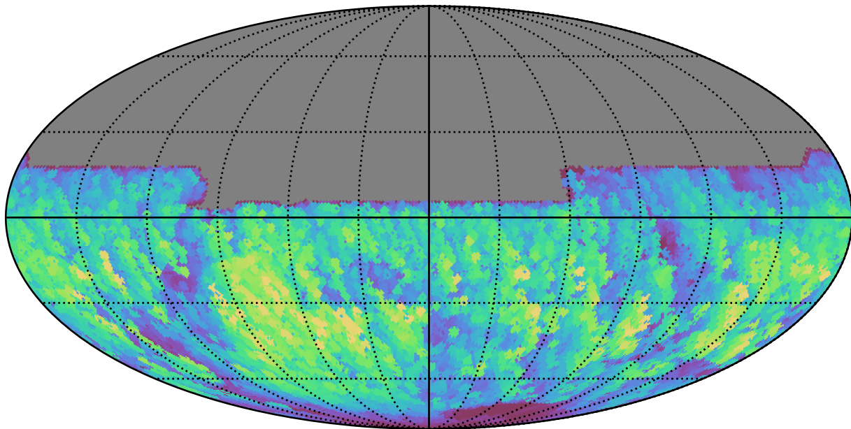
all_long_v3.4_10yrs All sky y band: Max normairmass
