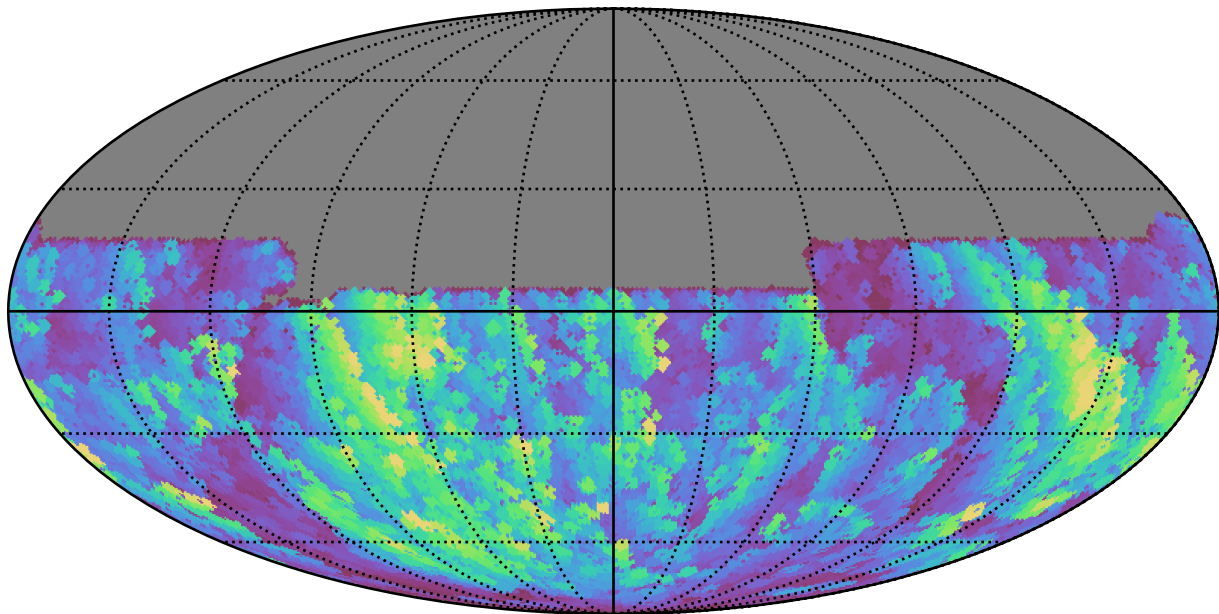
all_long_v3.4_10yrs All sky u band: Max normairmass
