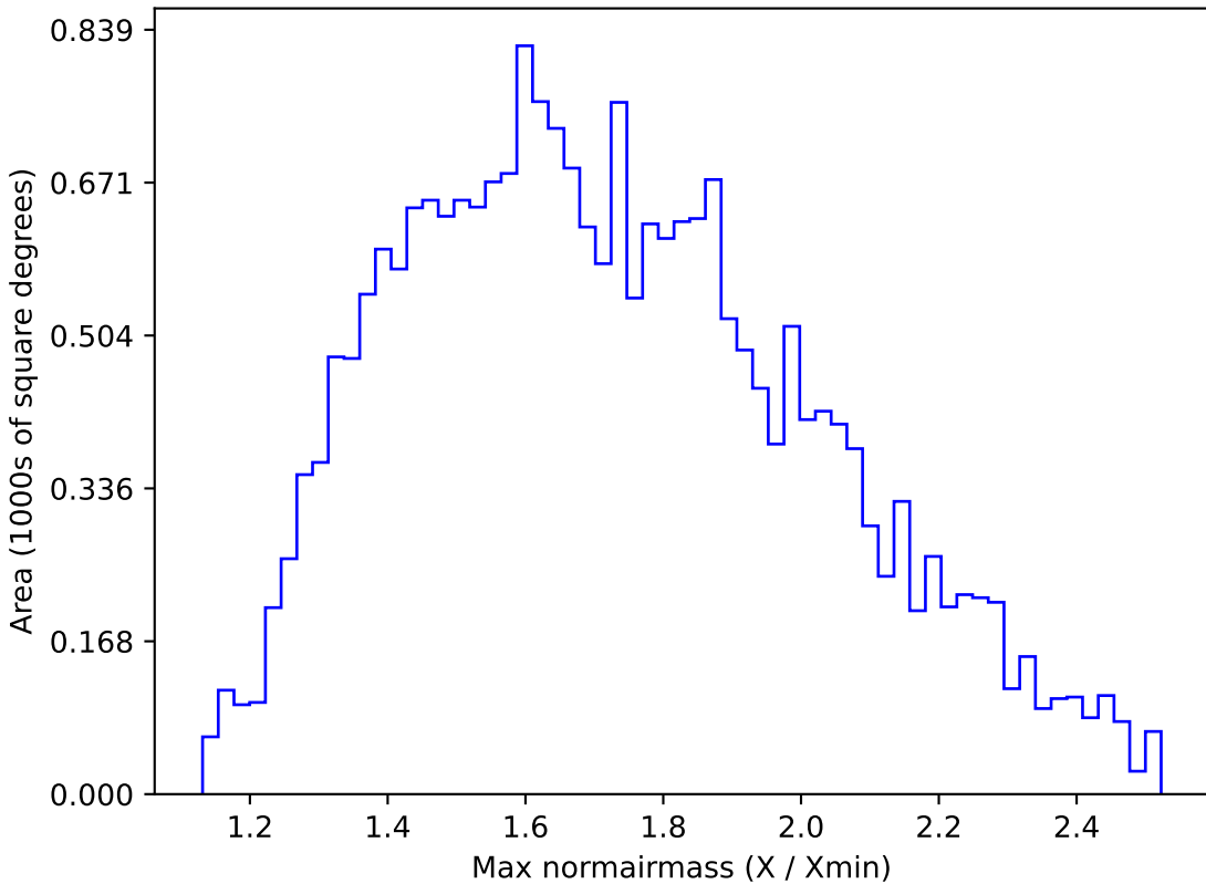
all_long_v3.4_10yrs All sky u band: Max normairmass
