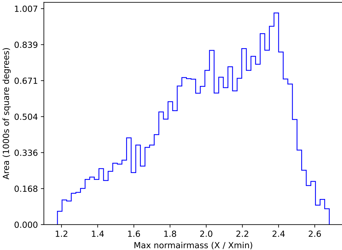
all_long_v3.4_10yrs All sky r band: Max normairmass
