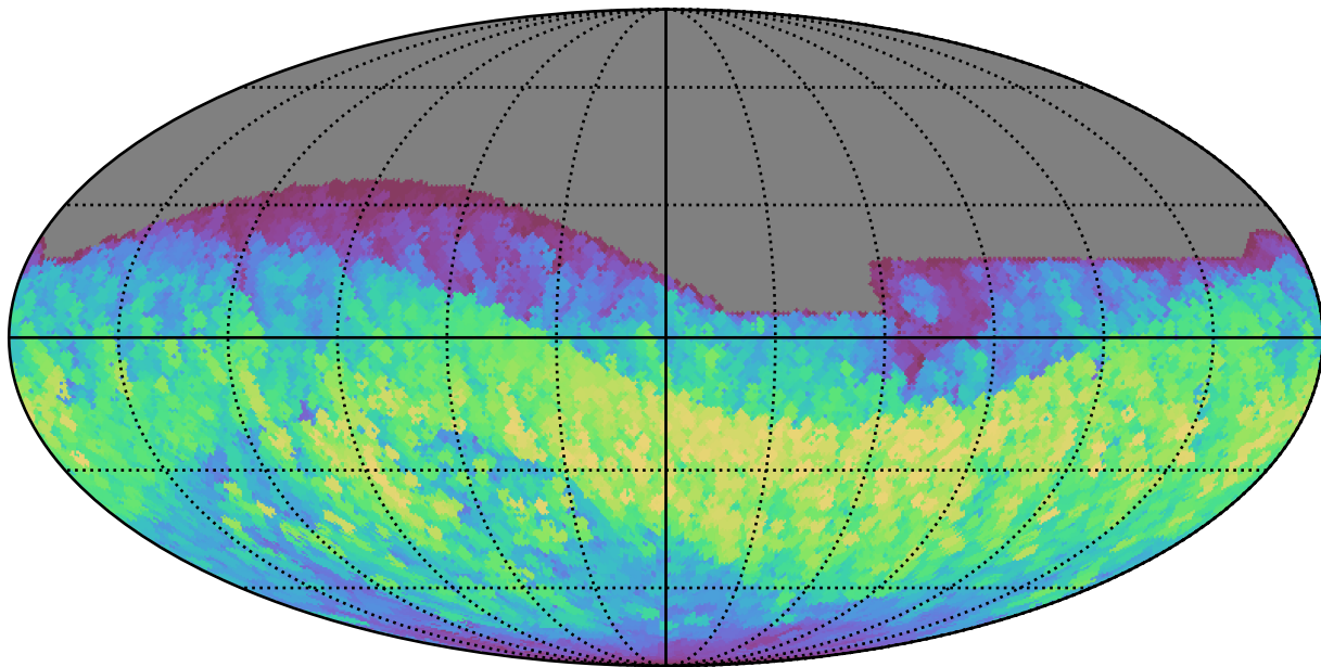
all_long_v3.4_10yrs All sky i band: Max normairmass
