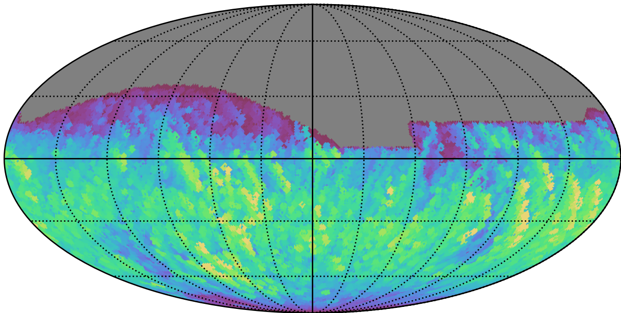
all_long_v3.4_10yrs All sky g band: Max normairmass
