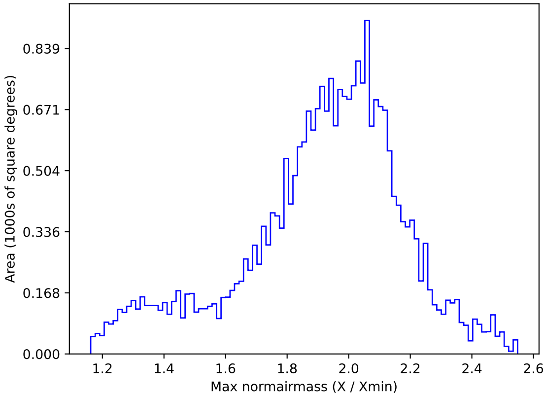
all_long_v3.4_10yrs All sky g band: Max normairmass
