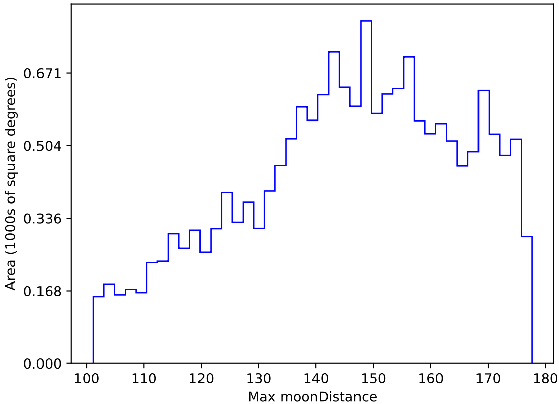
all_long_v3.4_10yrs WFD y band: Max moonDistance
