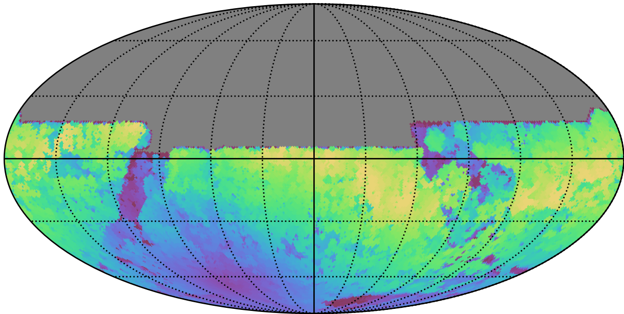
all_long_v3.4_10yrs All sky y band: Max moonDistance
