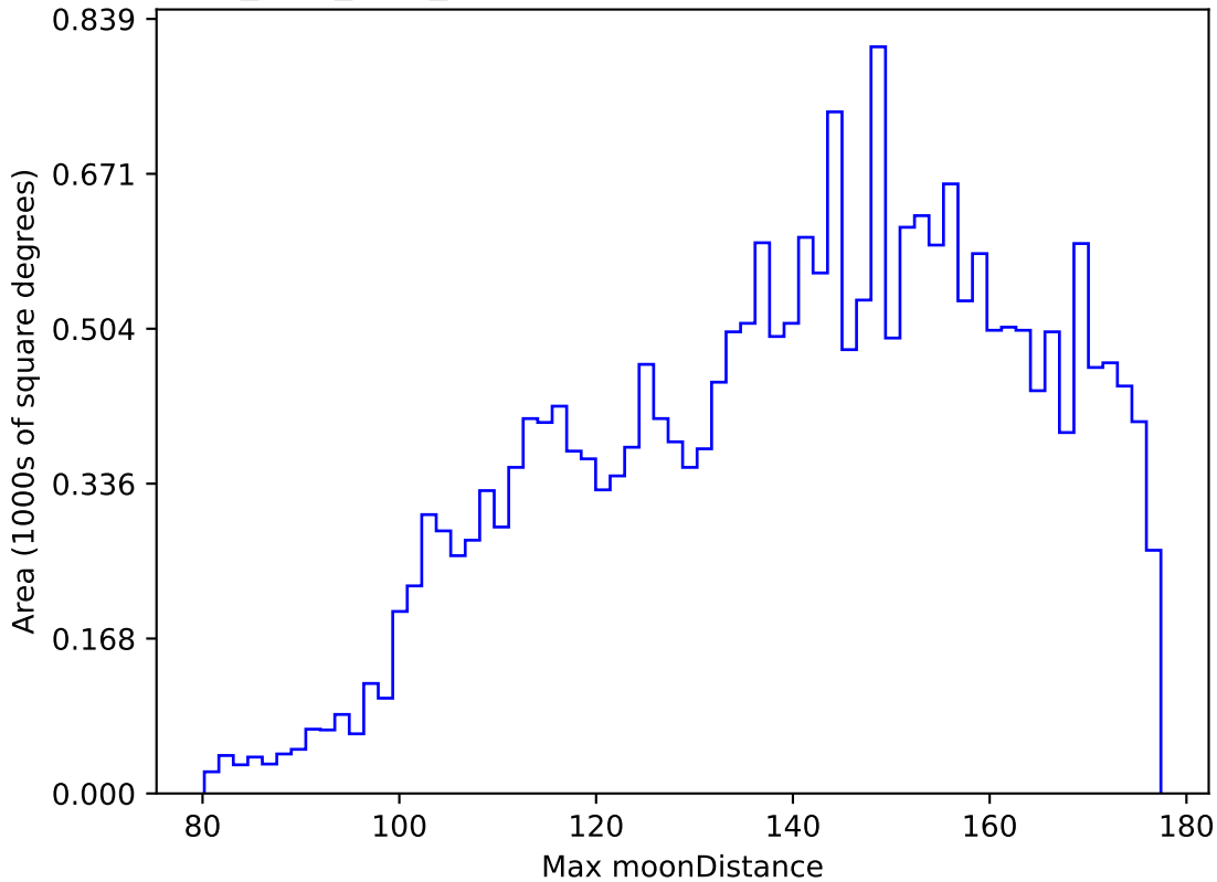
all_long_v3.4_10yrs All sky y band: Max moonDistance
