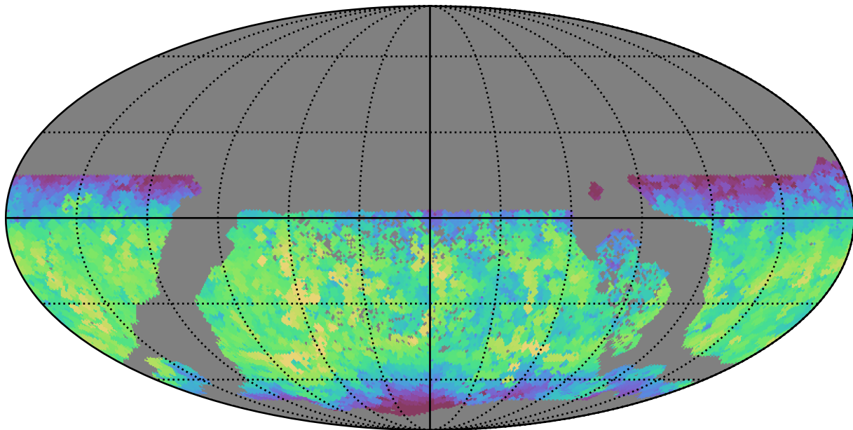
all_long_v3.4_10yrs WFD y band: Max fiveSigmaDepth
