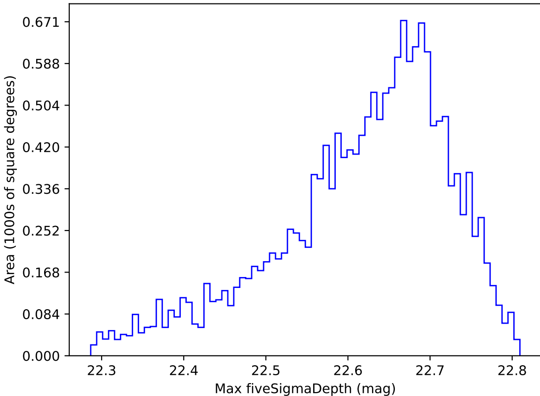
all_long_v3.4_10yrs WFD y band: Max fiveSigmaDepth
