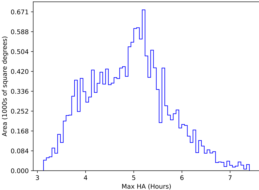
all_long_v3.4_10yrs WFD z band: Max HA
