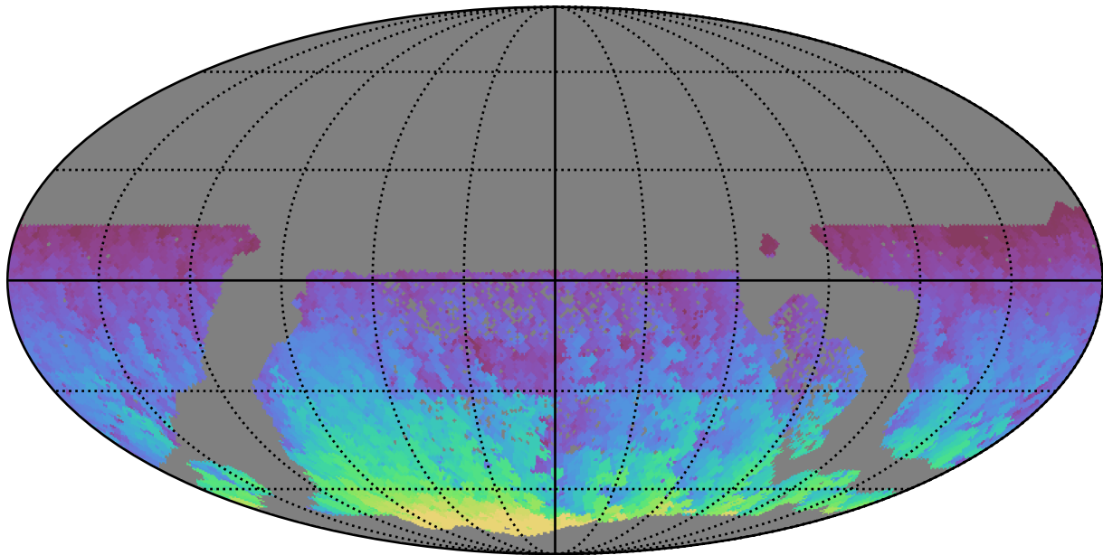
all_long_v3.4_10yrs WFD y band: Max HA
