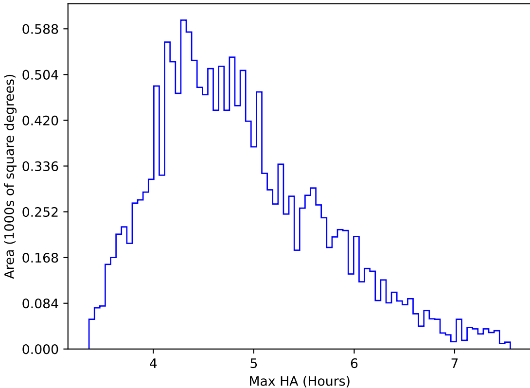
all_long_v3.4_10yrs WFD y band: Max HA
