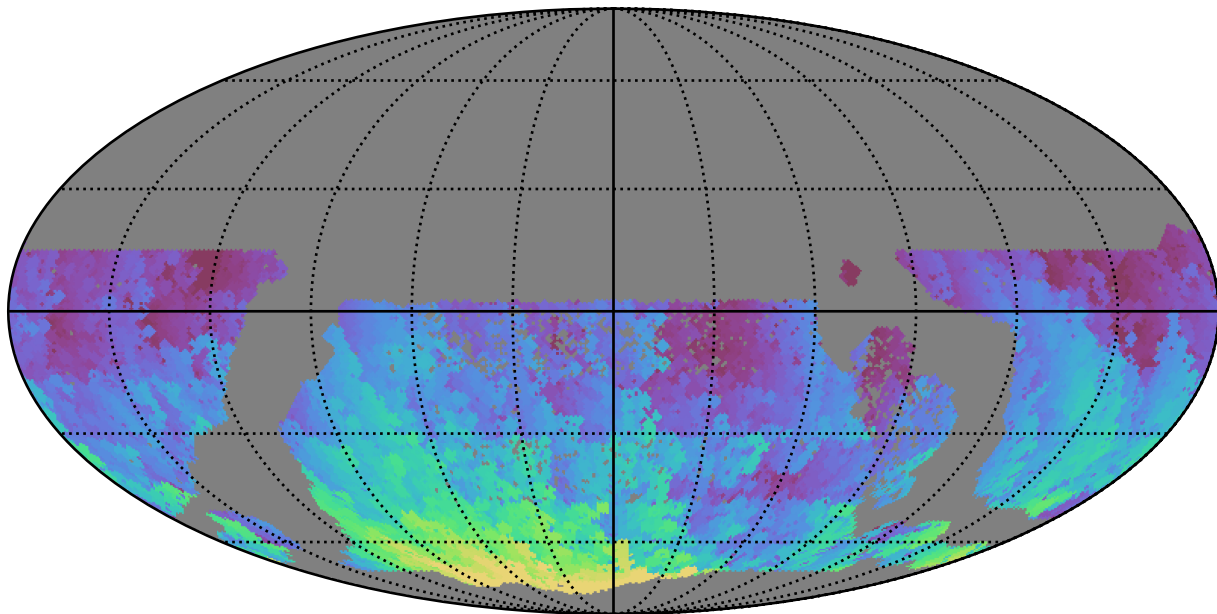
all_long_v3.4_10yrs WFD u band: Max HA
