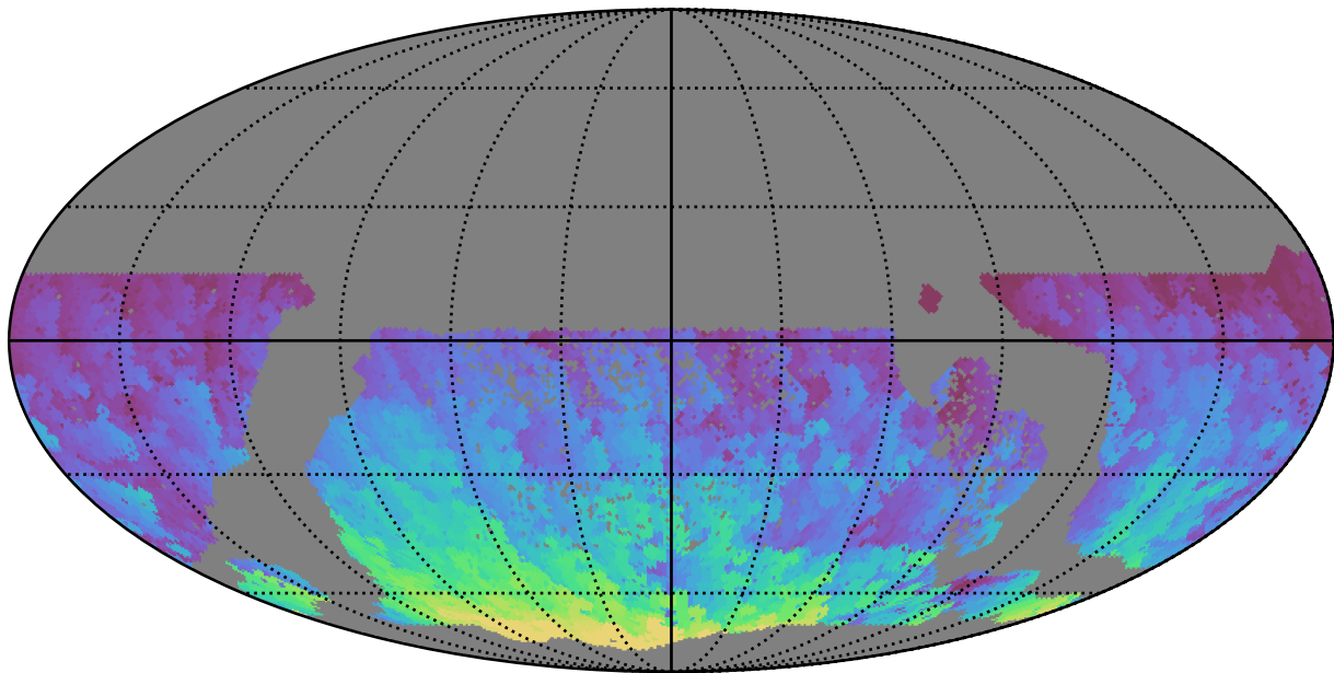
all_long_v3.4_10yrs WFD r band: Max HA
