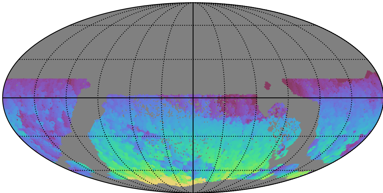
all_long_v3.4_10yrs WFD i band: Max HA
