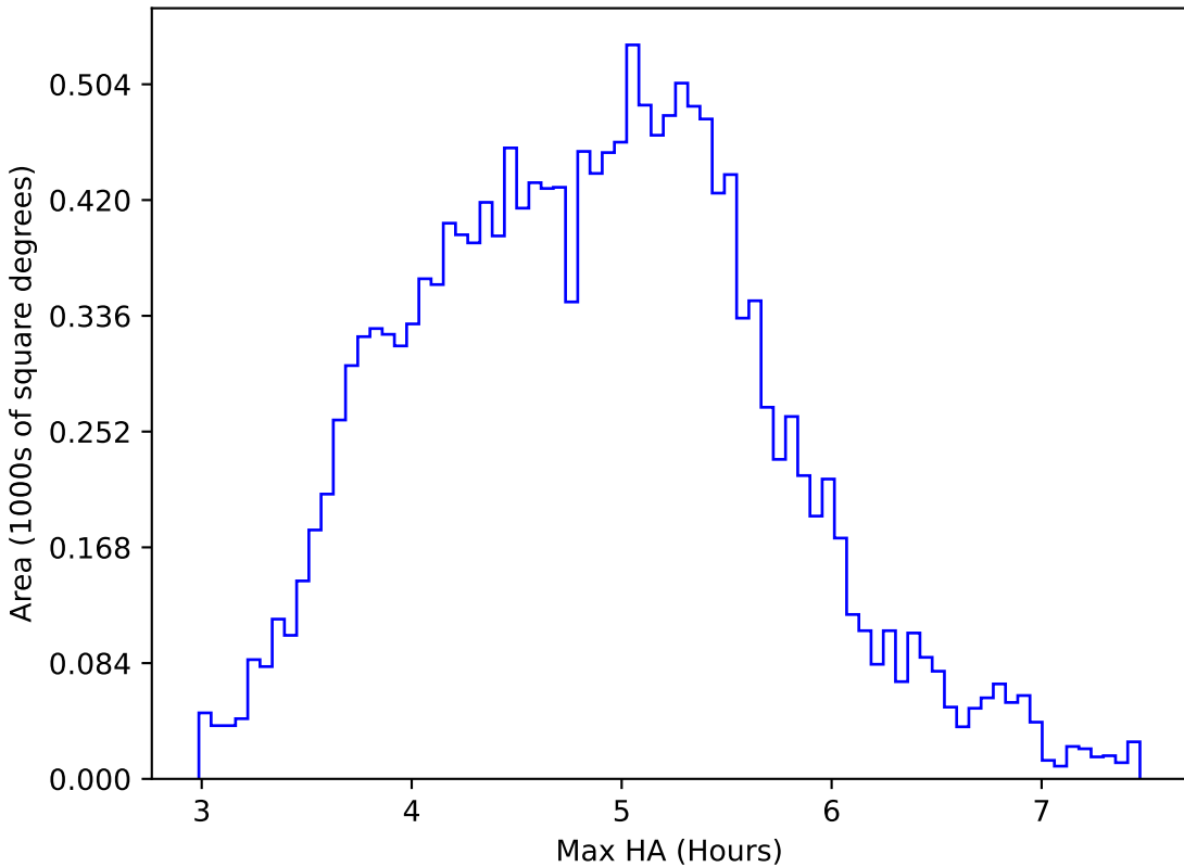
all_long_v3.4_10yrs WFD i band: Max HA
