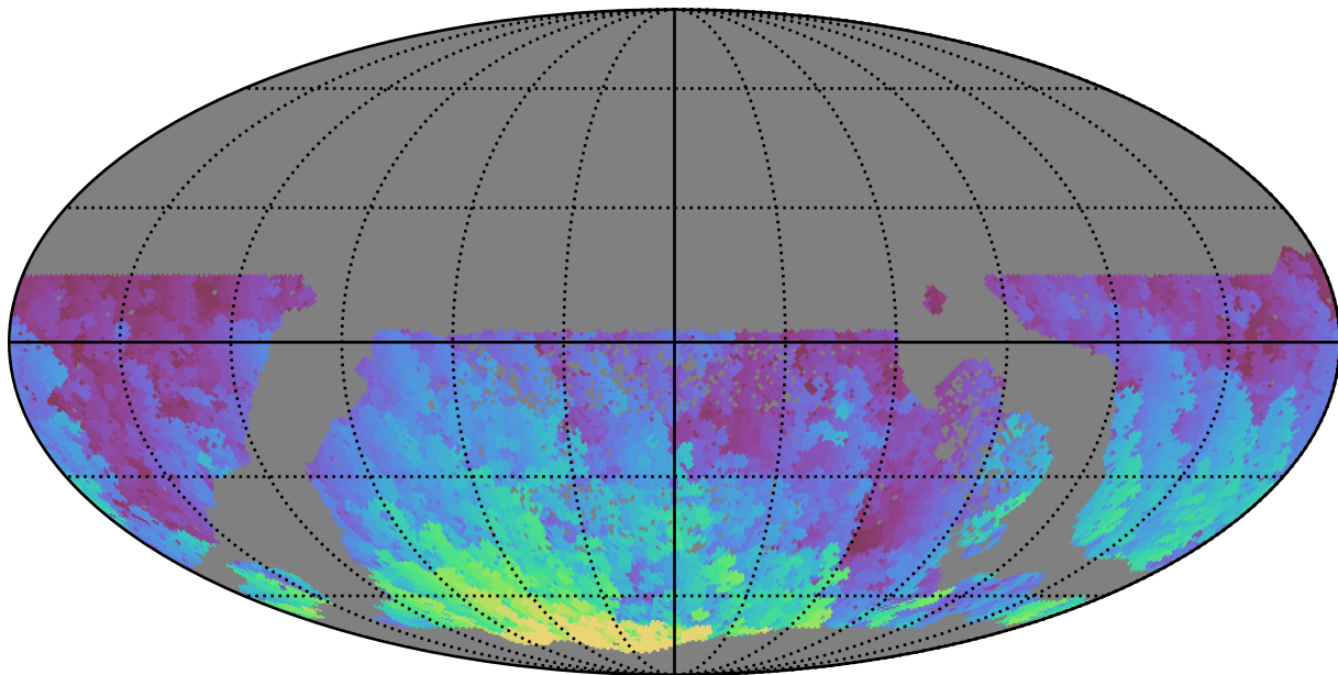
all_long_v3.4_10yrs WFD g band: Max HA
