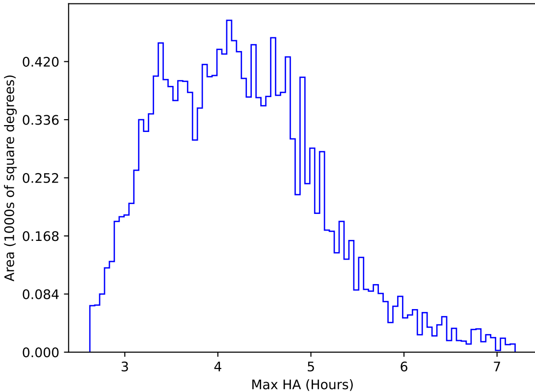
all_long_v3.4_10yrs WFD g band: Max HA
