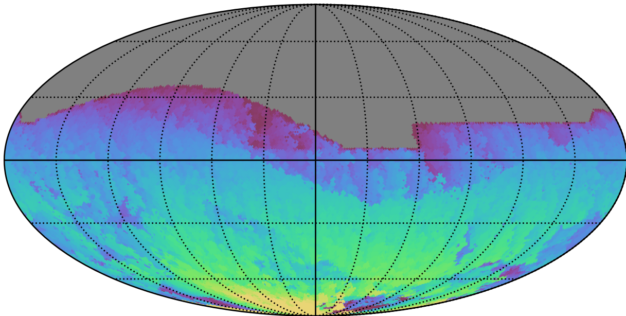
all_long_v3.4_10yrs All sky z band: Max HA
