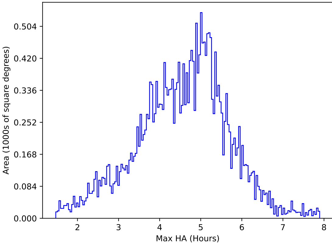
all_long_v3.4_10yrs All sky z band: Max HA
