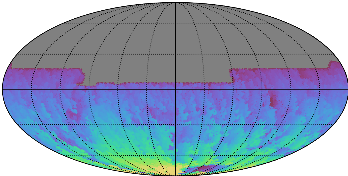
all_long_v3.4_10yrs All sky y band: Max HA
