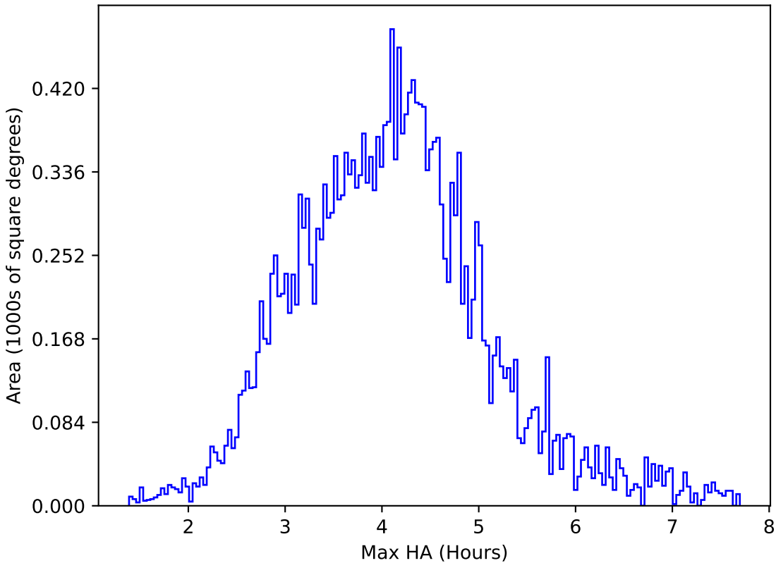
all_long_v3.4_10yrs All sky u band: Max HA
