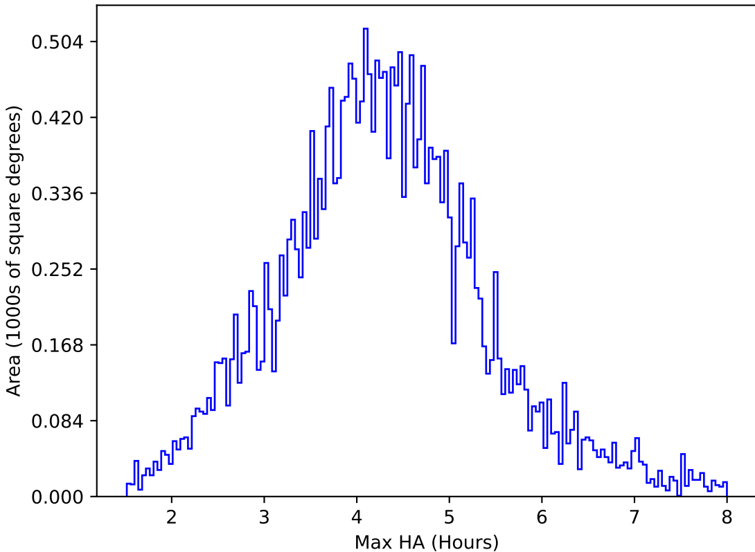
all_long_v3.4_10yrs All sky r band: Max HA
