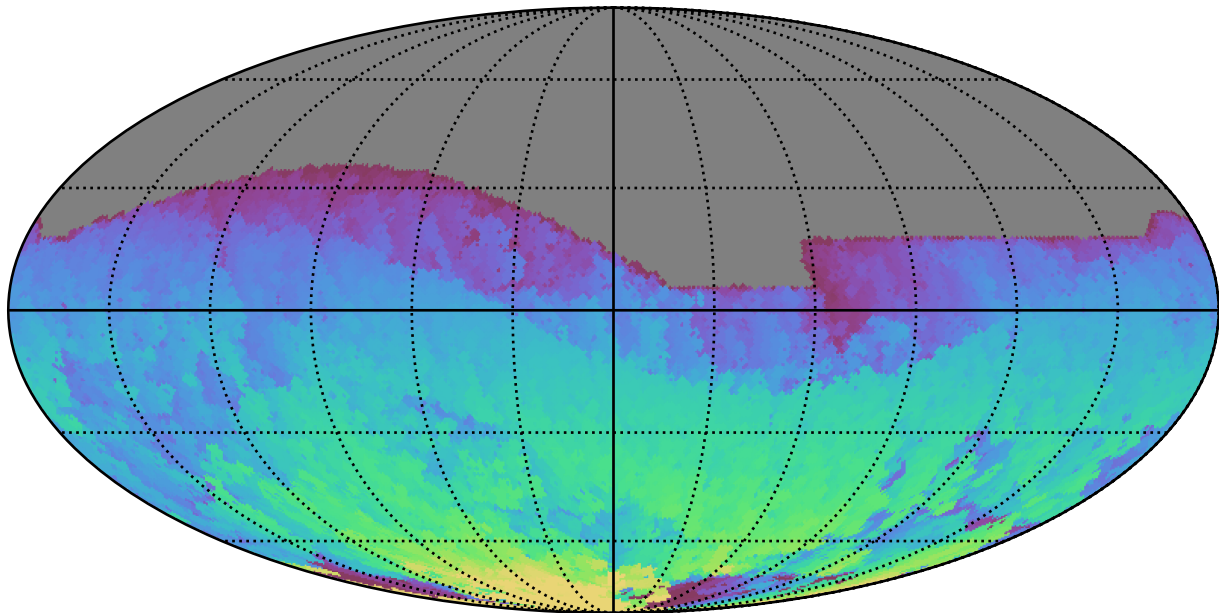
all_long_v3.4_10yrs All sky i band: Max HA
