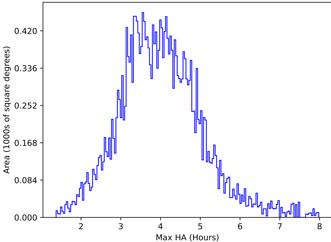
all_long_v3.4_10yrs All sky g band: Max HA
