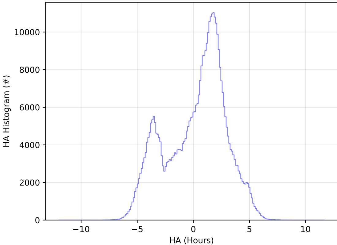
all_long_v3.4_10yrs WFD z band: HA Histogram
