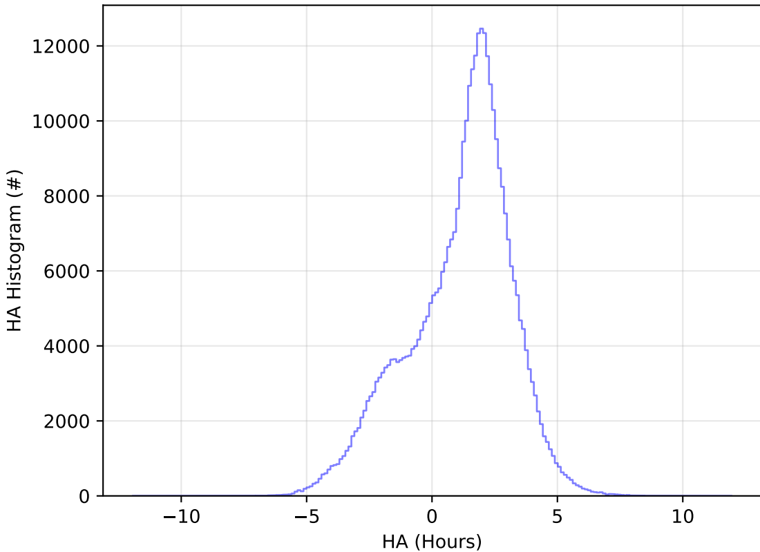
all_long_v3.4_10yrs All sky y band: HA Histogram
