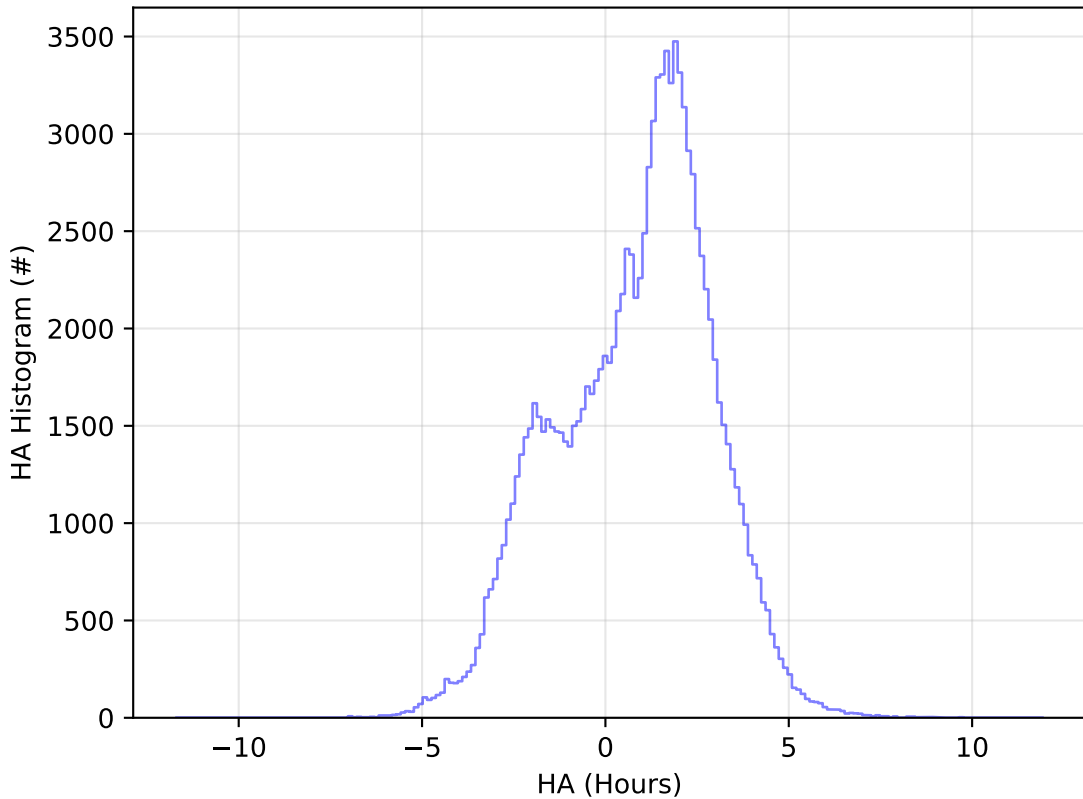
all_long_v3.4_10yrs All sky u band: HA Histogram
