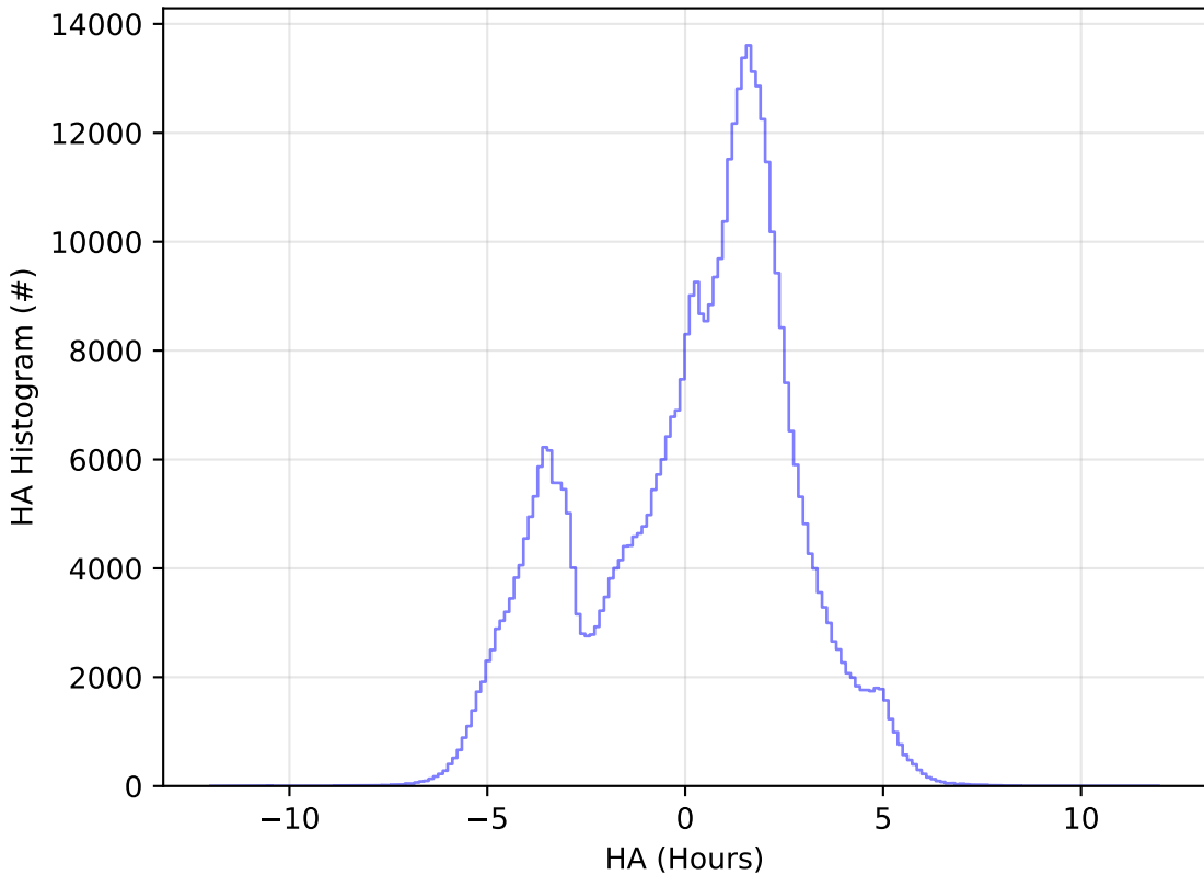
all_long_v3.4_10yrs All sky i band: HA Histogram
