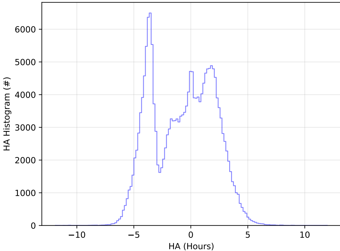
all_long_v3.4_10yrs All sky g band: HA Histogram
