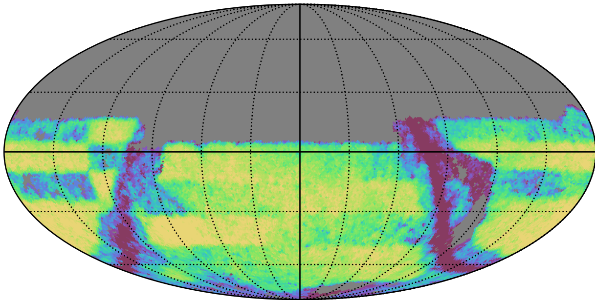
all_long_v3.4_10yrs Yr 3-4 y band: Exgal_CoaddM5
