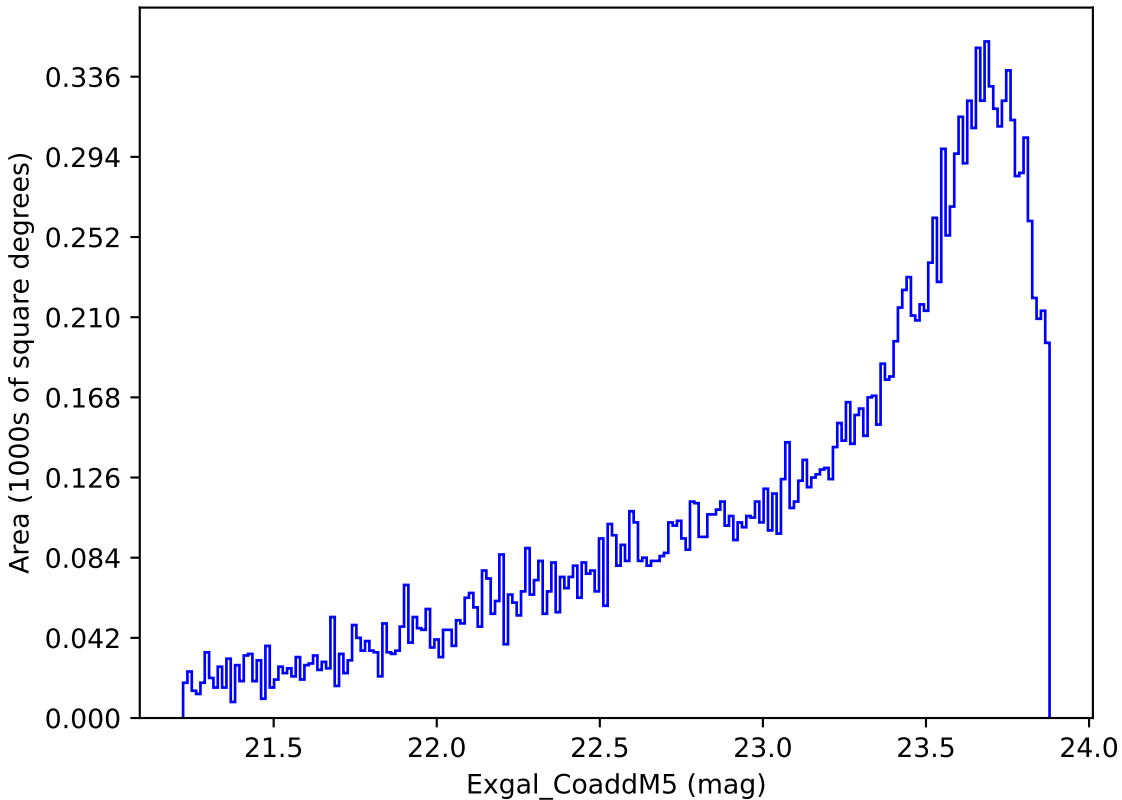
all_long_v3.4_10yrs Yr 3-4 y band: Exgal_CoaddM5
