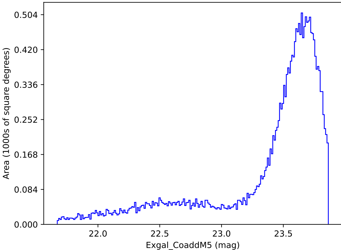
all_long_v3.4_10yrs Yr 1 y band: Exgal_CoaddM5
