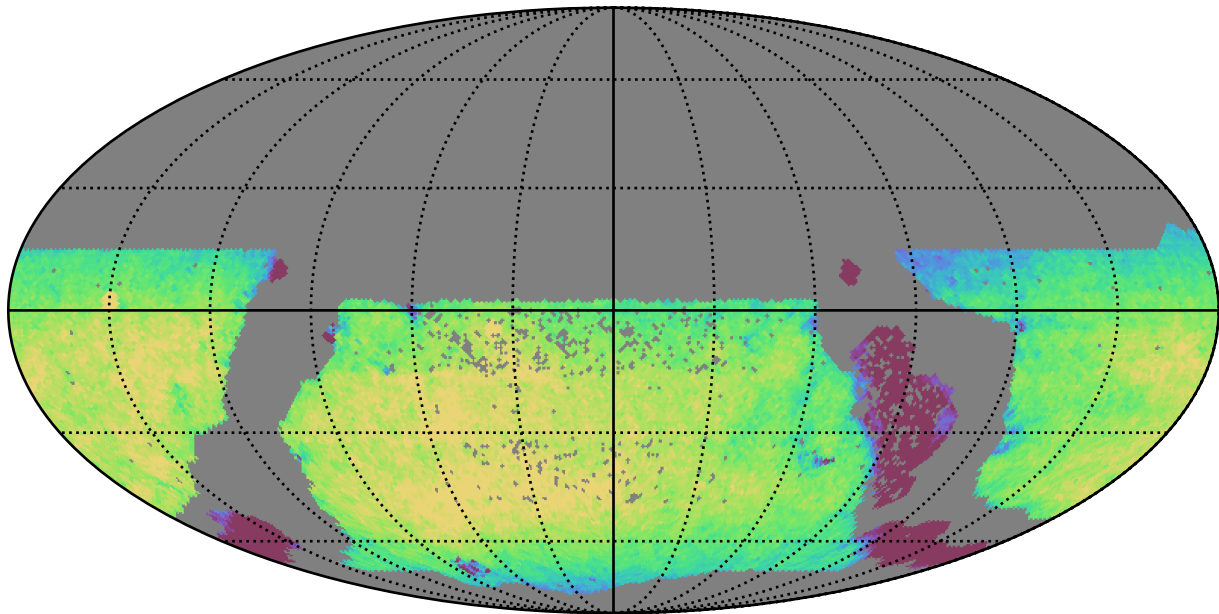
all_long_v3.4_10yrs WFD y band: Exgal_CoaddM5
