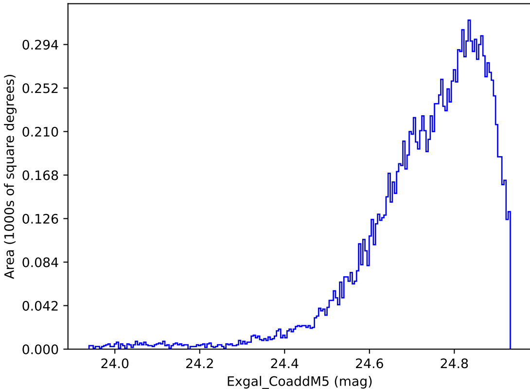
all_long_v3.4_10yrs WFD y band: Exgal_CoaddM5
