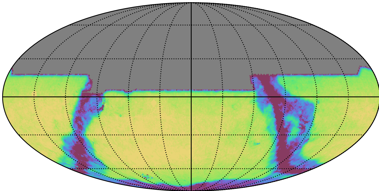
all_long_v3.4_10yrs All sky y band: Exgal_CoaddM5
