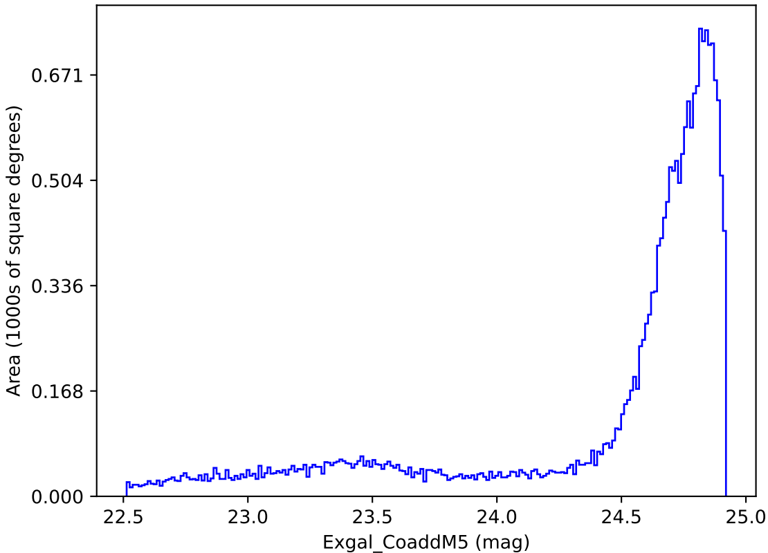
all_long_v3.4_10yrs All sky y band: Exgal_CoaddM5
