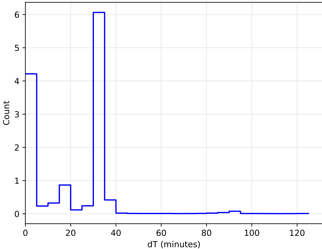
all_long_v3.4_10yrs All sky: DeltaT Histogram
