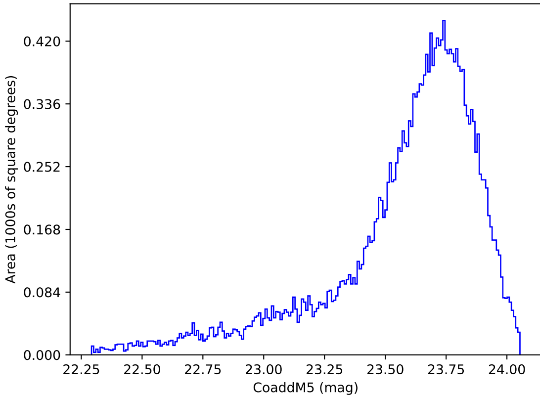
all_long_v3.4_10yrs Yr 1 y band: CoaddM5
