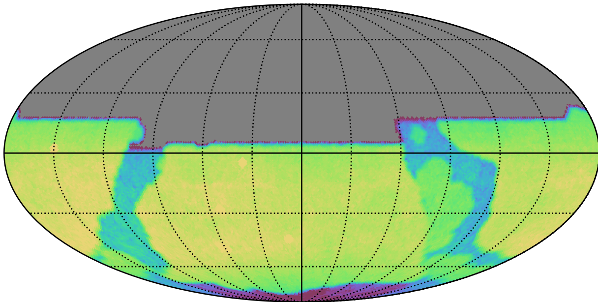
all_long_v3.4_10yrs All sky y band: CoaddM5
