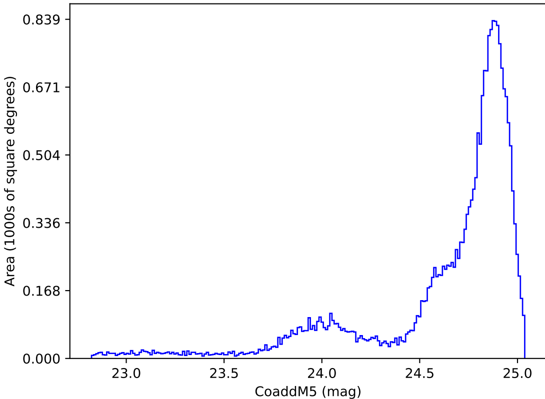
all_long_v3.4_10yrs All sky y band: CoaddM5
