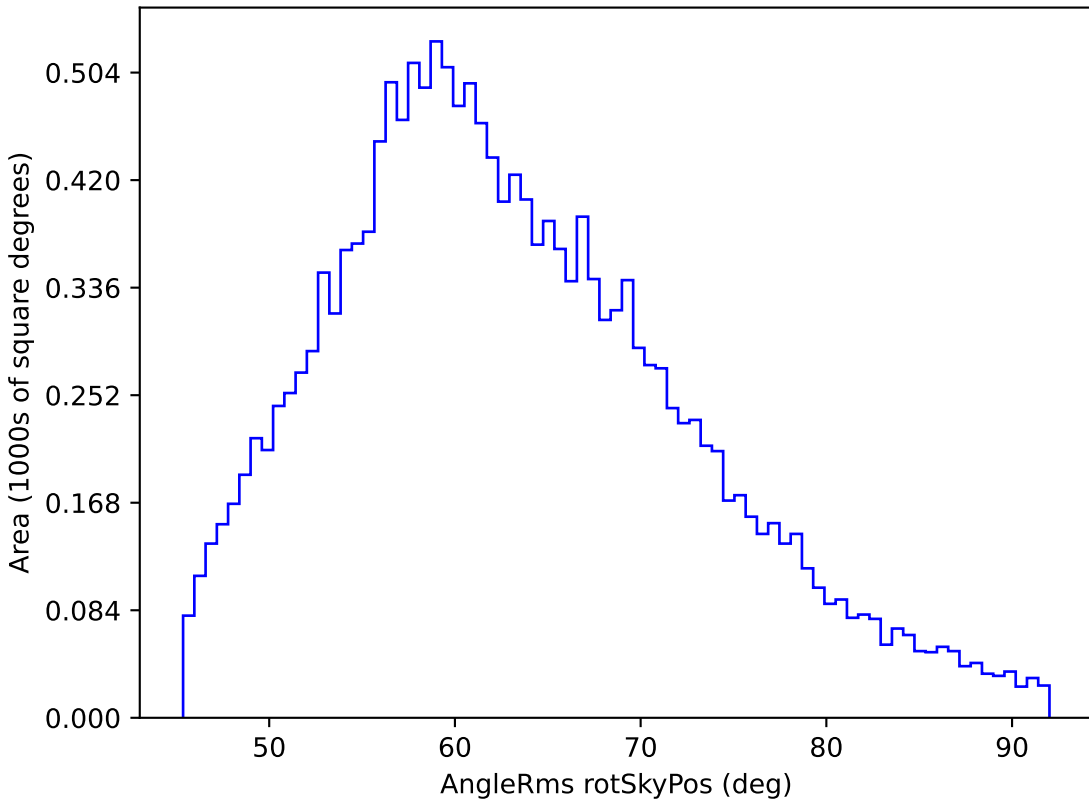
all_long_v3.4_10yrs WFD y band: AngleRms rotSkyPos
